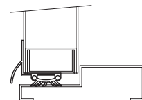
B-SILL
