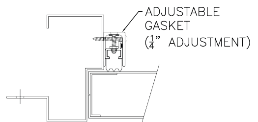
JAMB SECTION
